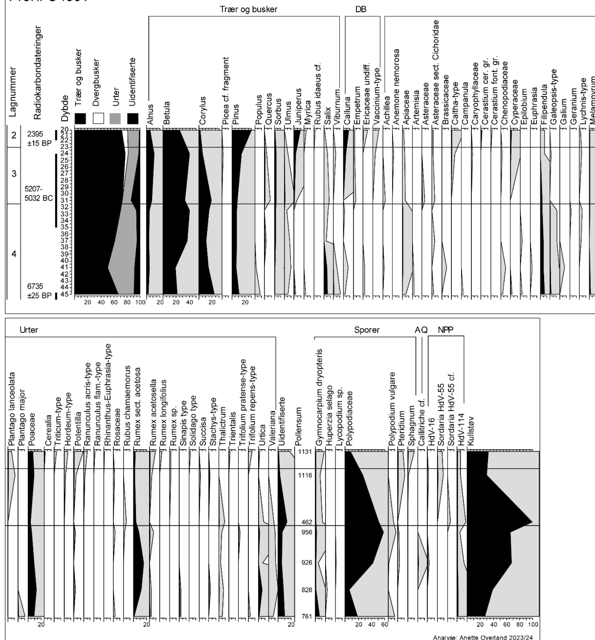
Figure 3. Pollendiagram (%) fra lokalitet 4, profil C4301. Sorte kurver viser prosent, og grå skygge viser 20x forstørrelse for å synliggjøre lave prosentverdier.
